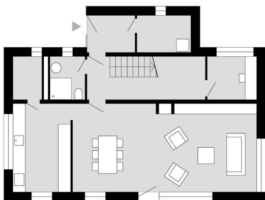
+ půdorys přízemí
